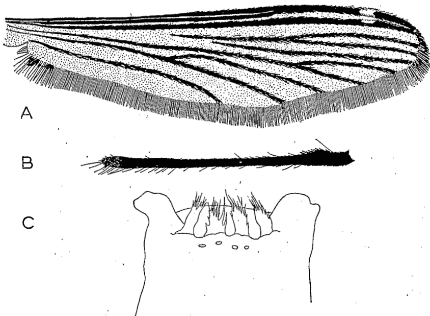
Fig. 1. — Anopheles caroni .
